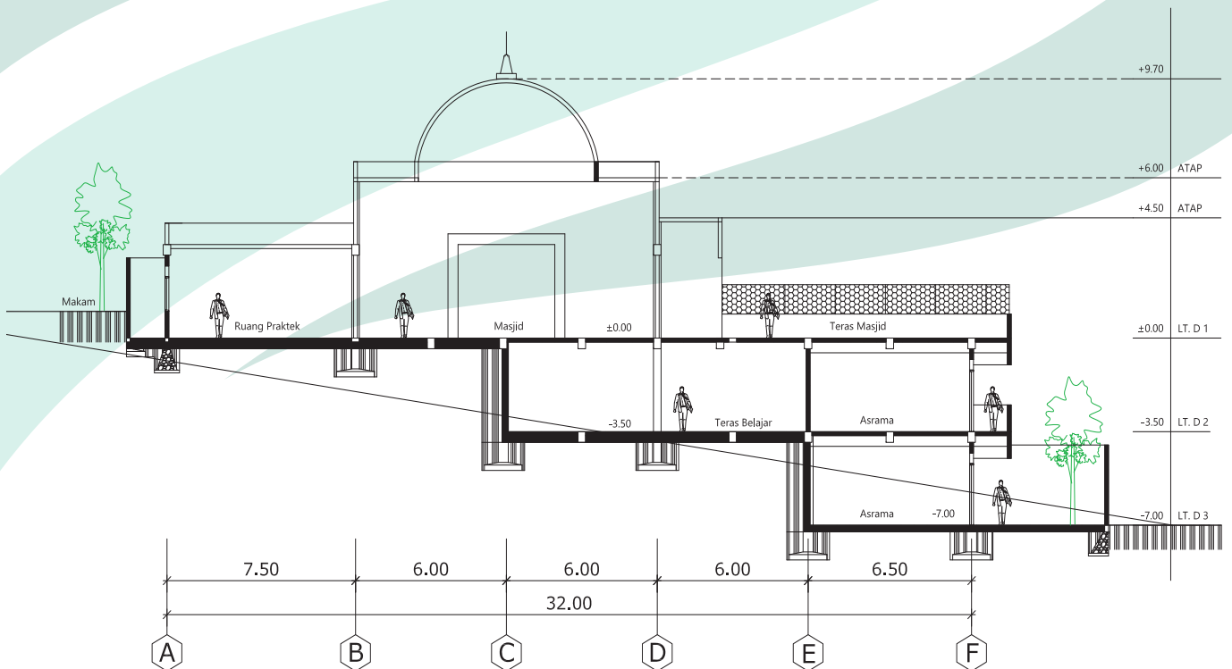
POTONGAN 3-3 SKALA 1 : 100
